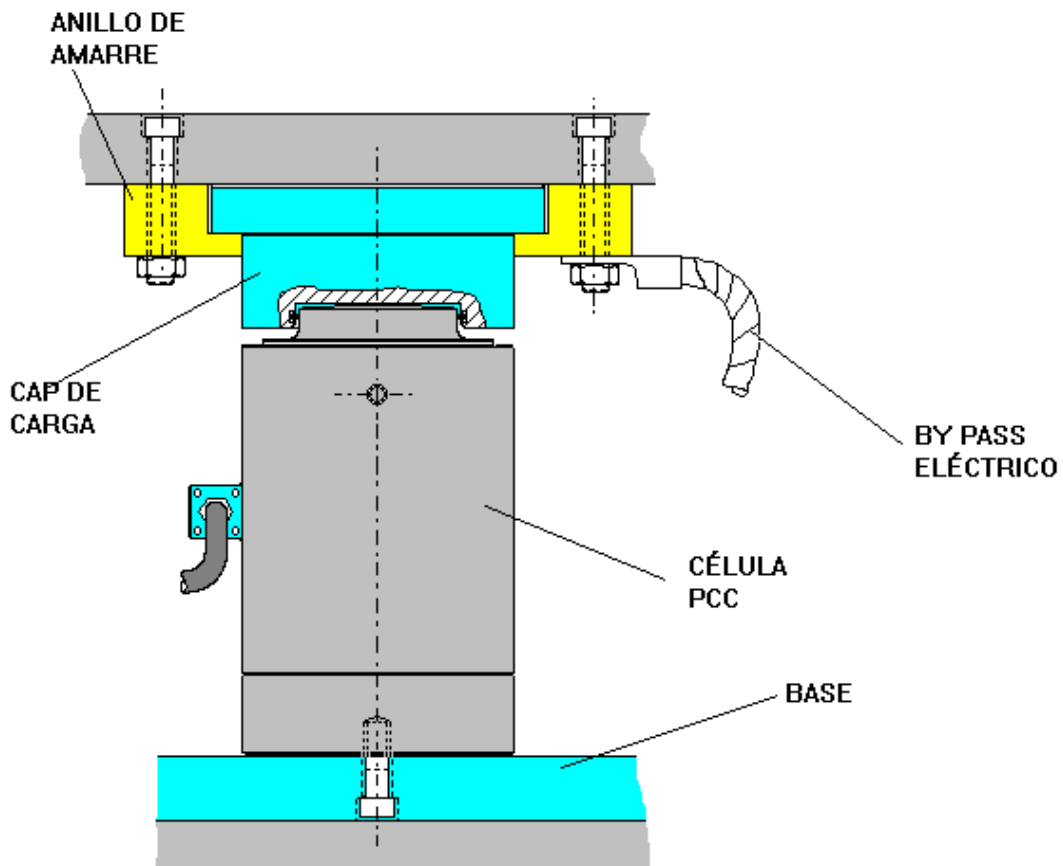
MONTAJE DE CÉLULA DE CARGA PCC CON CONJUNTO CM/PCC-2
